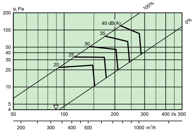
ROC 400 + ALS 315-400, Extract air
