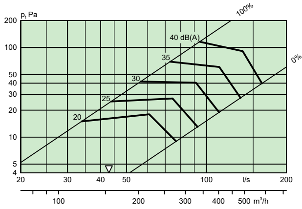
ROC 250 + ALS 200-250, Extract air
