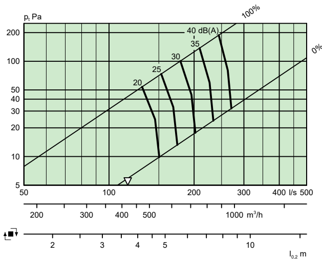
ROC 400 + ALS 315-400, Supply air
